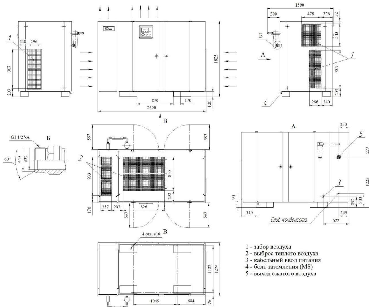
Установка компрессорная ВК60P-Д. Установочные и присоединительные размеры.
